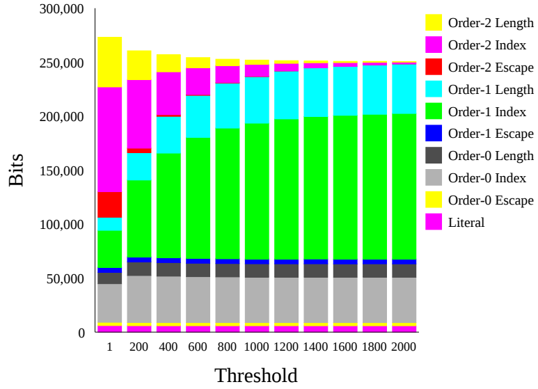
(d) Order-2 LZ77-PM
